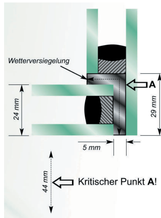
Abb. 7 Fehlerhafte Fugentiefe bei 1 K-Dichtstoff
