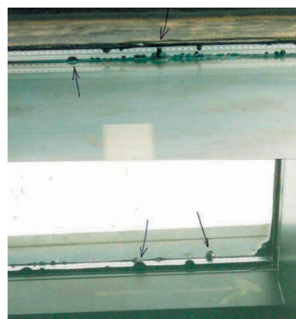
Abb. 2 Auflösen der Butyl-Dichtung durch Migration
